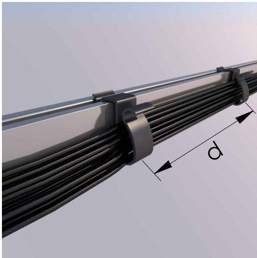
**Installazione a pressione nella guida profilata.
