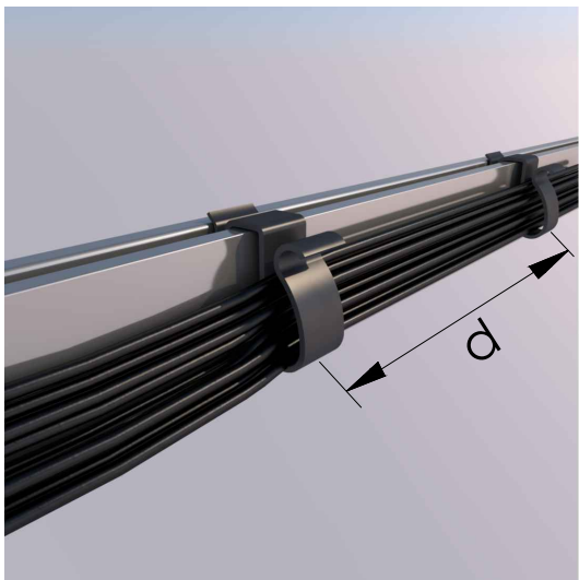
**Instalación mediante presión en el carril del perfil.
