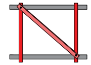
Arriostamiento para 2 triángulos
