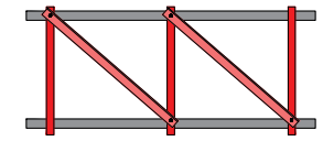
Arriostamiento para 3 triángulos
