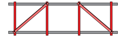
Arriostamiento para 4 o más triángulos
